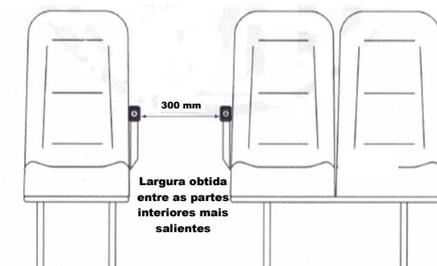
Figura 14 – Largura mínima do corredor de circulação
