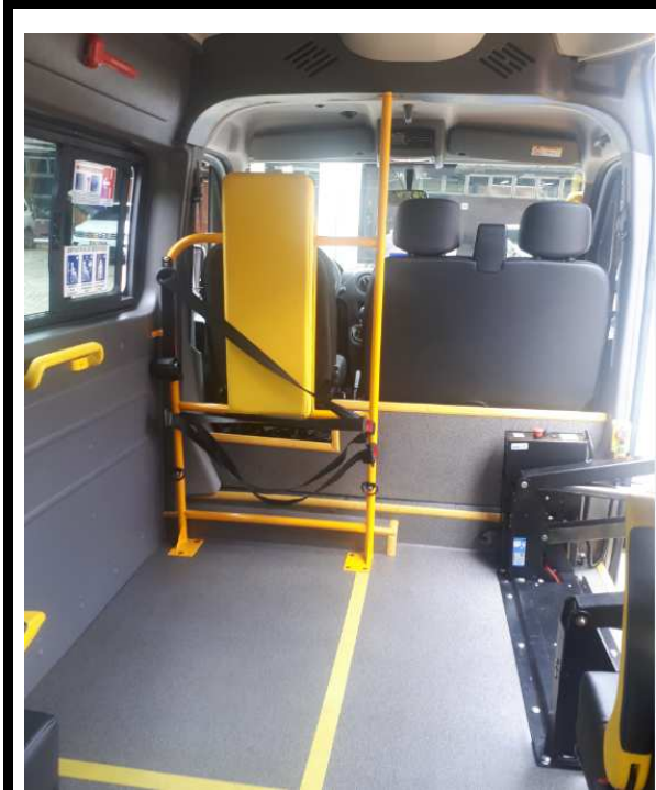
A área livre em frente à entrada (área de manobra) permite o giro da cadeira e o deslocamento para
