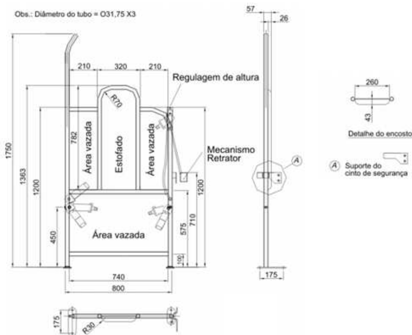
Figura 11 – Guarda-corpo
