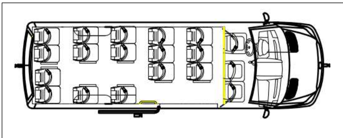
4B – Veículo com poltronas individualizadas e corredor central
