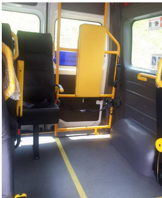
Área do cadeirante posicionada no sentido longitudinal e em direção à marcha do veículo
