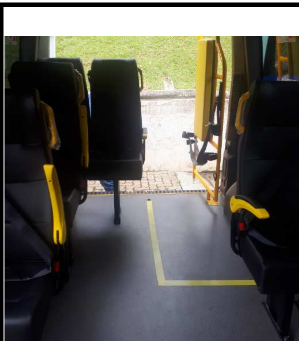
Salão de passageiros misto, com área reservada para cadeira de rodas e bancos individualizados
