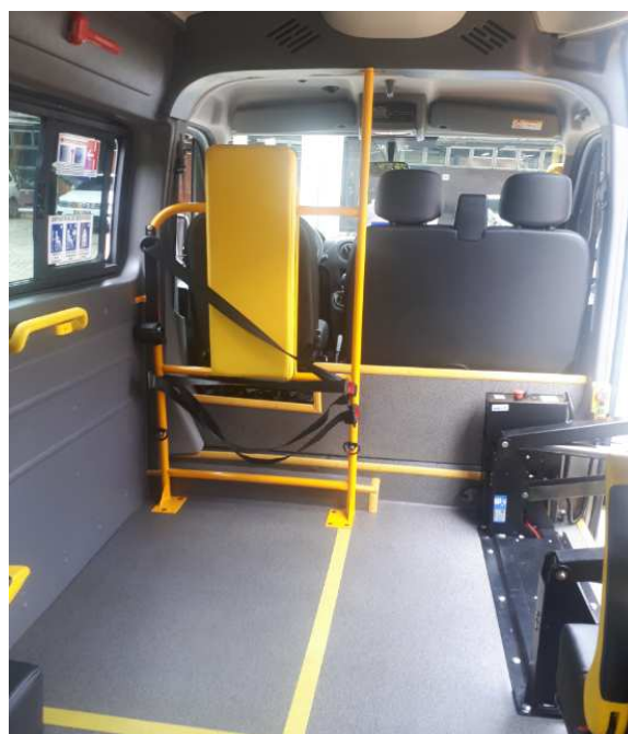
Área do cadeirante posicionada no sentido longitudinal e em direção contrária à marcha do veículo
