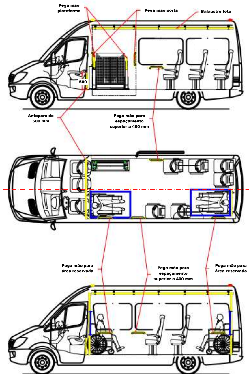
Figura 17 – Pontos de apoio e anteparos
