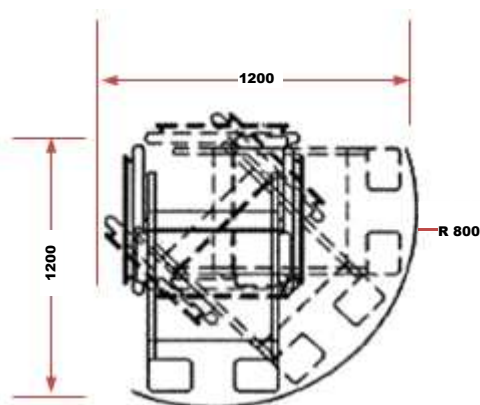
Figura 10 – Área de giro para manobra
